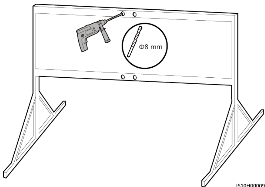
Figura 4-14 Perfuração
